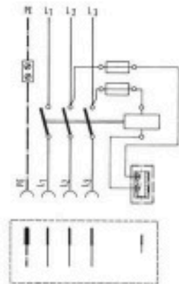
PSK - vergrendeling
