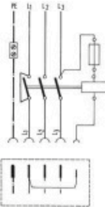
Conventionele vergrendeling
